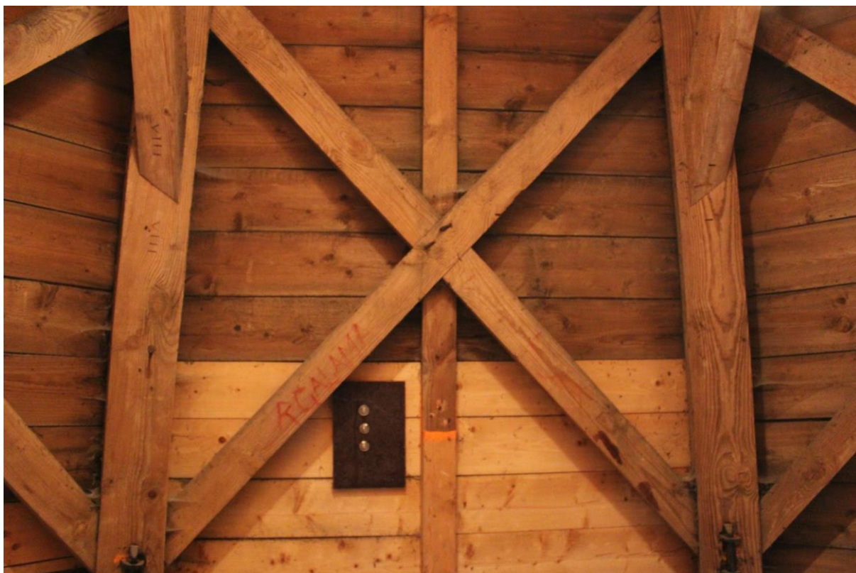
Foto 32. Een deel van de torenspits met een andreaskruis tussen twee hoekkepers. OP de aansluiting van de korbelen met de hoekkepers zijn gehakte telmerken zichtbaar. Rechts een gehakte I en links een gehakte VIII.
